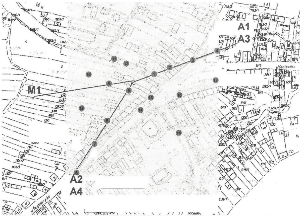
Azymuty anten T-Mobile
