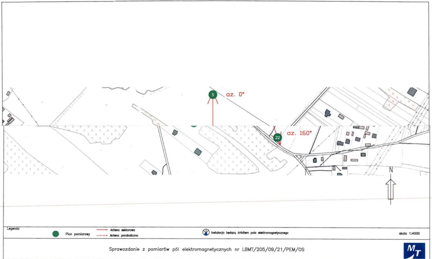
Rys.1 Lokalizacja pionów pomiarowych
